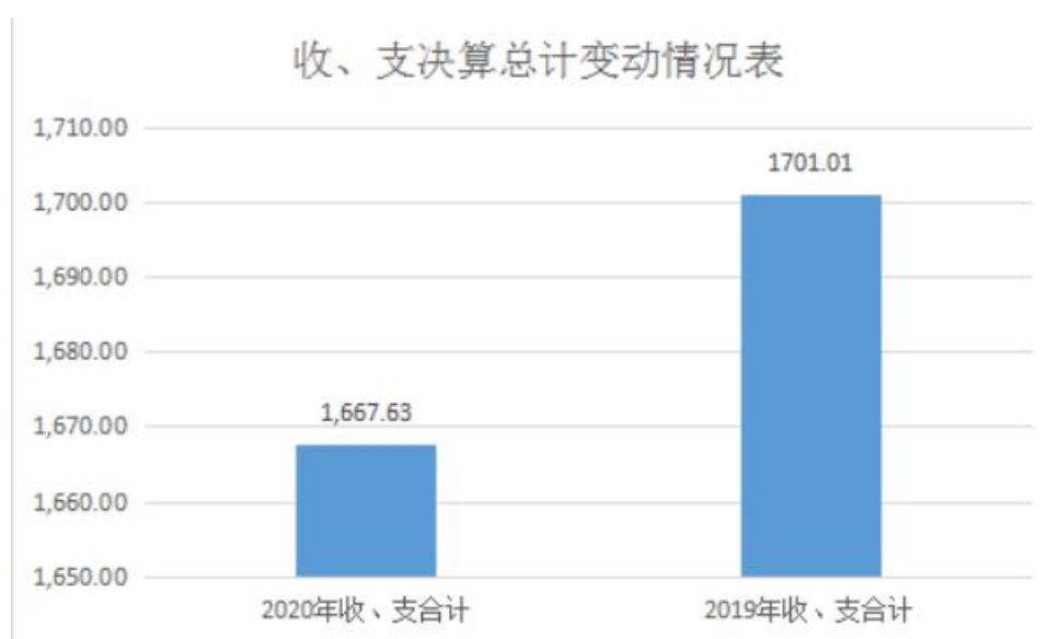
图 1：收、支决算总计变动情况表 单位：万元
